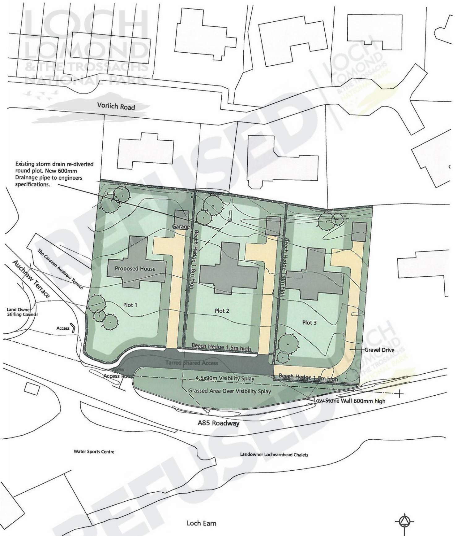
Site Plan 1:500
