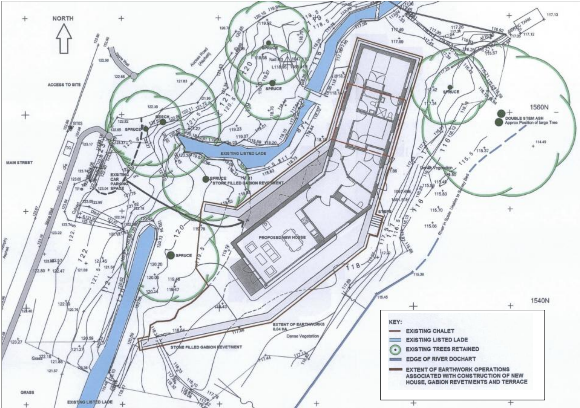
Appendix 5 Site Plan
